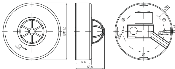
Рисунок 3 – Габаритные размеры
